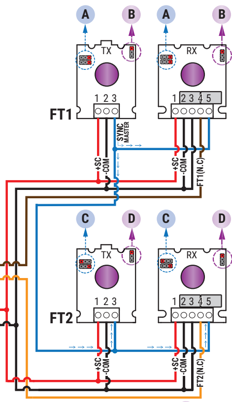
JUMPER DI SINCRONIZZAZIONE (PER MASTER) SYNCHRONISATION JUMPER (FOR MASTER)
